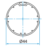
A3505_0515 Adapter & Mitnehmer Rundrohr Filtersun 44
