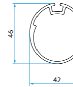
A3505_0508 Adapter & Mitnehmer Oval 42x46
