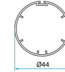
A3505_0507 Adapter & Mitnehmer Delfin 44 und Acmeda 44
